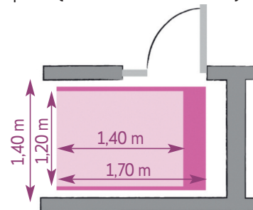
Cas de portes battantes ouverture en poussant
